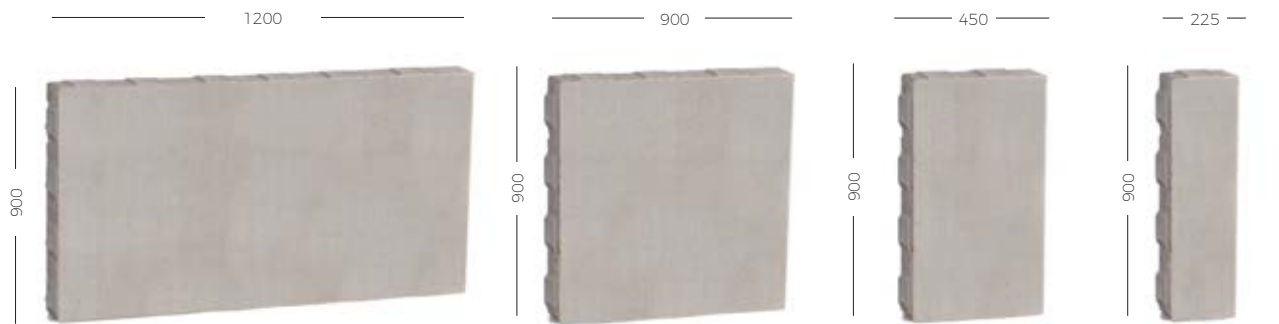
Paleta 16 1200 x 900 x 80 mm Paleta 1 900 x 900 x 80 mm Paleta 2 450 x 900 x 80 mm Paleta 3 900 x 225 x 80 mm
